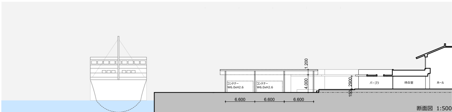
断面図 1:500
